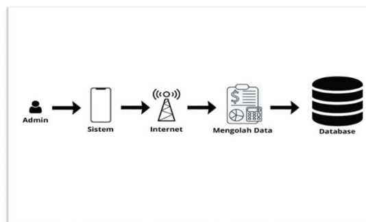
Gambar 1. Arsitektur Model
