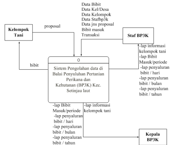
Gambar 3. Context Diagram Sistem Informasi
